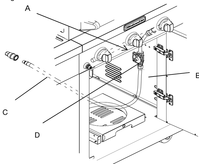
A. Tubulure de distribution B. Panneau de droite C. Tuyau à gaz en PVC de 10 pi (3 m) D. Ensemble détendeur pour gaz naturel/tuyau
